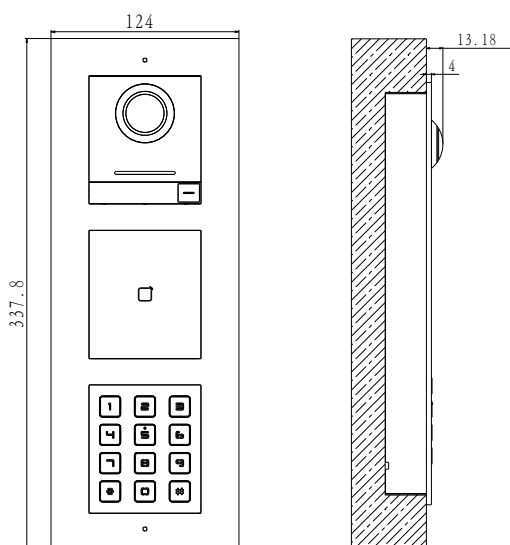
Montage encastré de trois modules
