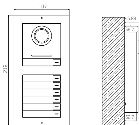
Montage en surface de deux modules
