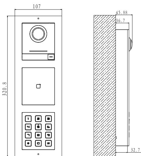
Montage en surface de trois modules
