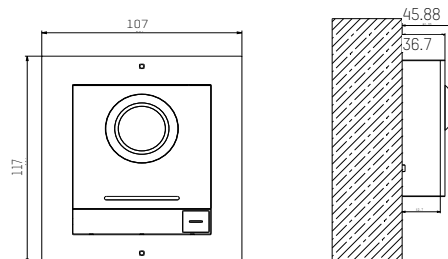
Montage en surface de module unique
