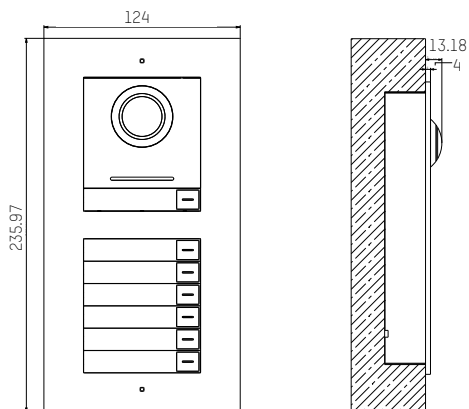
Montage encastré de deux modules
